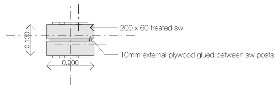
C01 AXO PLAN SCALE: 1:10
