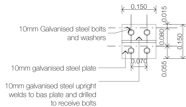
C01 AXO BASE PLAN SCALE: 1:10
