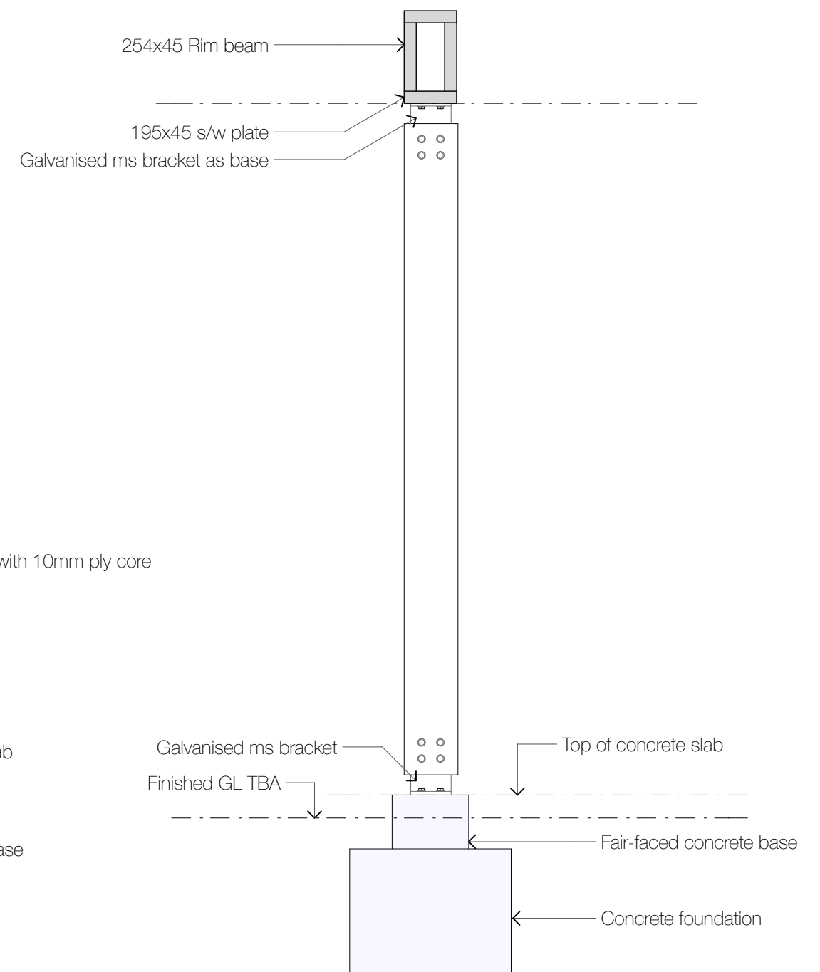
C01 AXO SIDE ELE SCALE: 1:20
