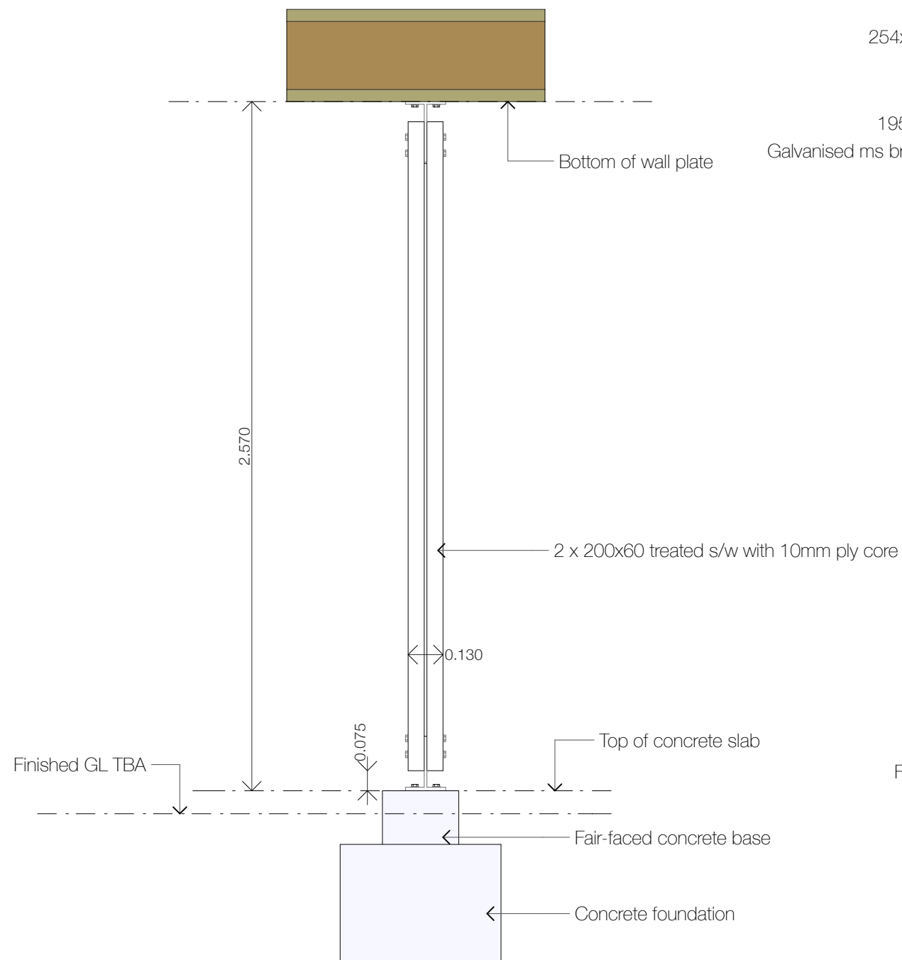
C01 AXO FRONT ELE SCALE: 1:20
