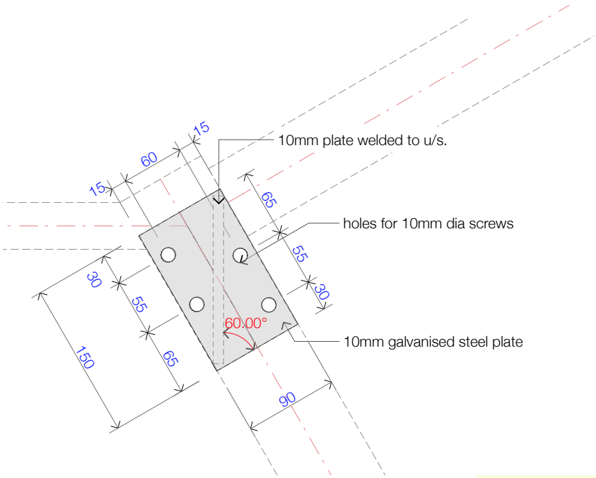
C06 PLAN top Plate SCALE: 1:5
